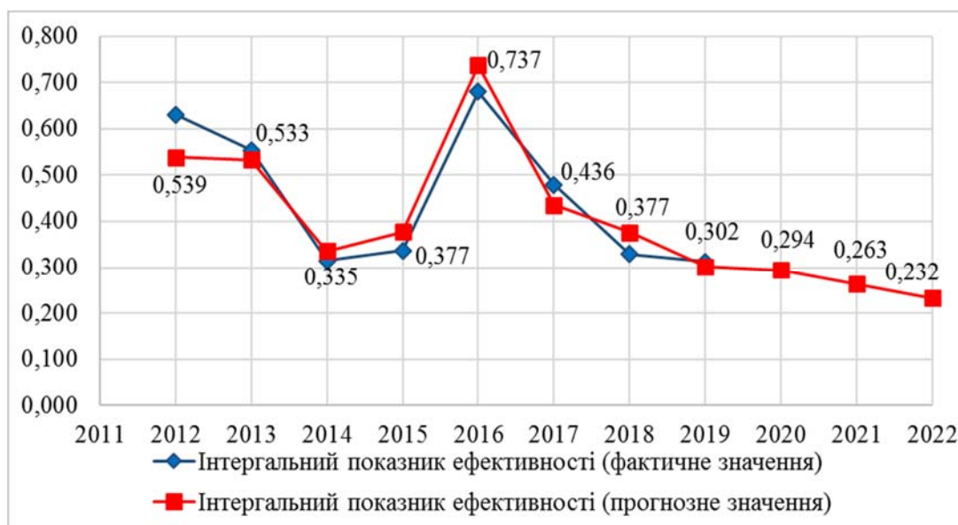
Рис. 2. Динаміка прогнозного значення інтегрального показника ефективності електродвигуна АІР 80 ПАТ «Харківський електротехнічний завод «Укрелектромаш»»
