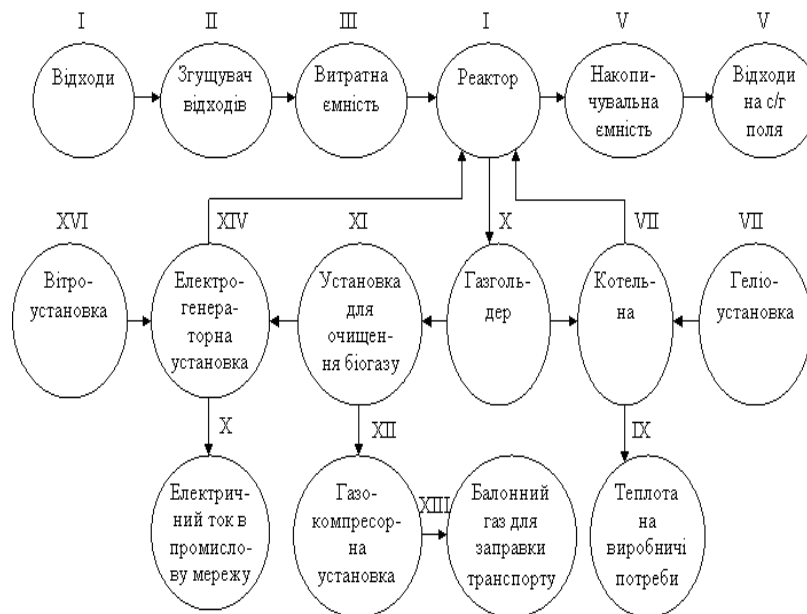
Рис. 2. Схема енергокомплексу з біогазовою установкою і газокompресорною станцією для крупних сільськогосподарських підприємств
