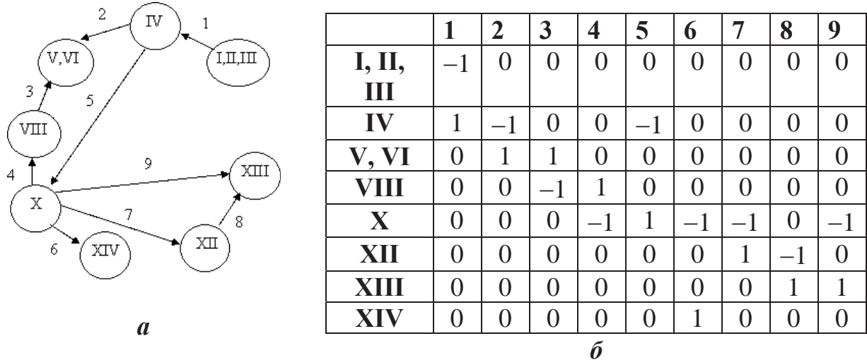
Рис. 4. Матеріальний потоковий граф (а) і матриця інцидентій схеми БГУ згідно рис. 2 (б).
