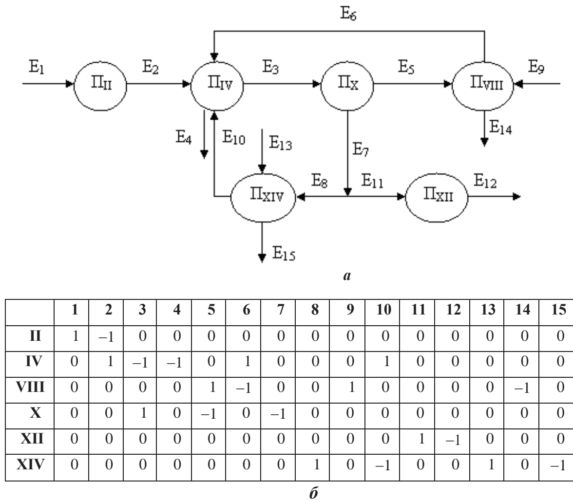
Рис. 5. Ексергетичний потоковий граф (а) і відповідна матриця інцидентій схеми по рис. 2 (б)
