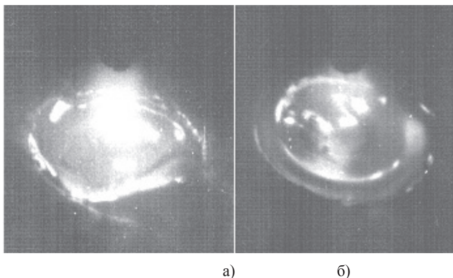
Рис. 1. Фрагменты скоростной киносъемки процессов протекающих в зоне сварки: V_{св} = 7\text{ мм/с} ; I_{св} = 170\text{ А} ; скорость съемки – 500 кадр/с; а) – B = 0 ; б) – B = 2 \cdot 10^{-2}\text{ Т}
